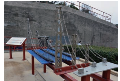
図11 ゴールデンゲート・ブリッジにあったエクスペラトリウム提供の実験装置。吊り橋の塔が高いほど張力が弱くてすむ。
