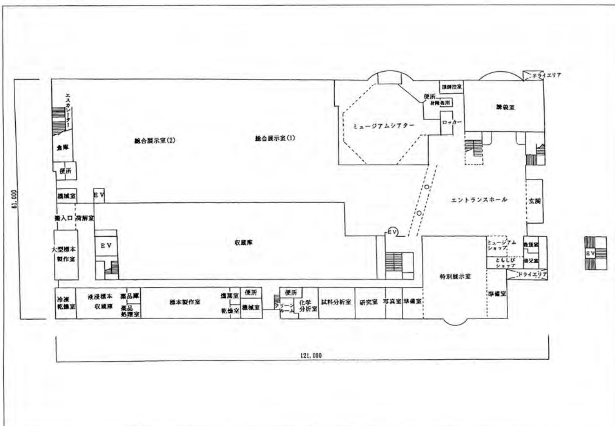
〔1階平面図〕
