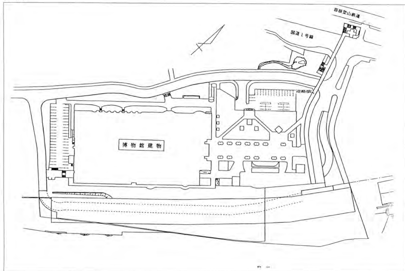
配置図
