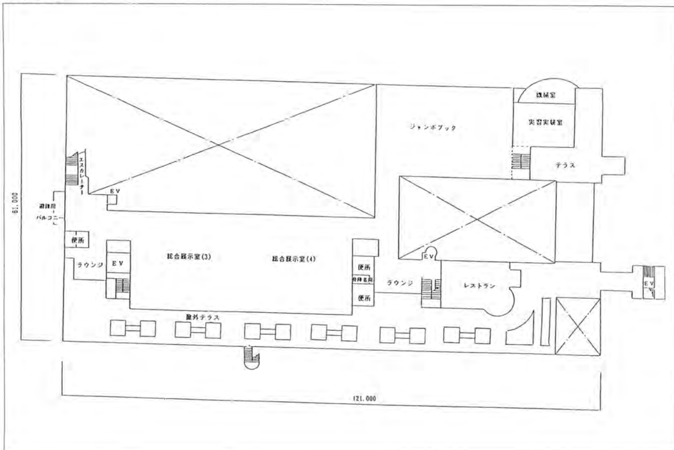
3 階平面図
