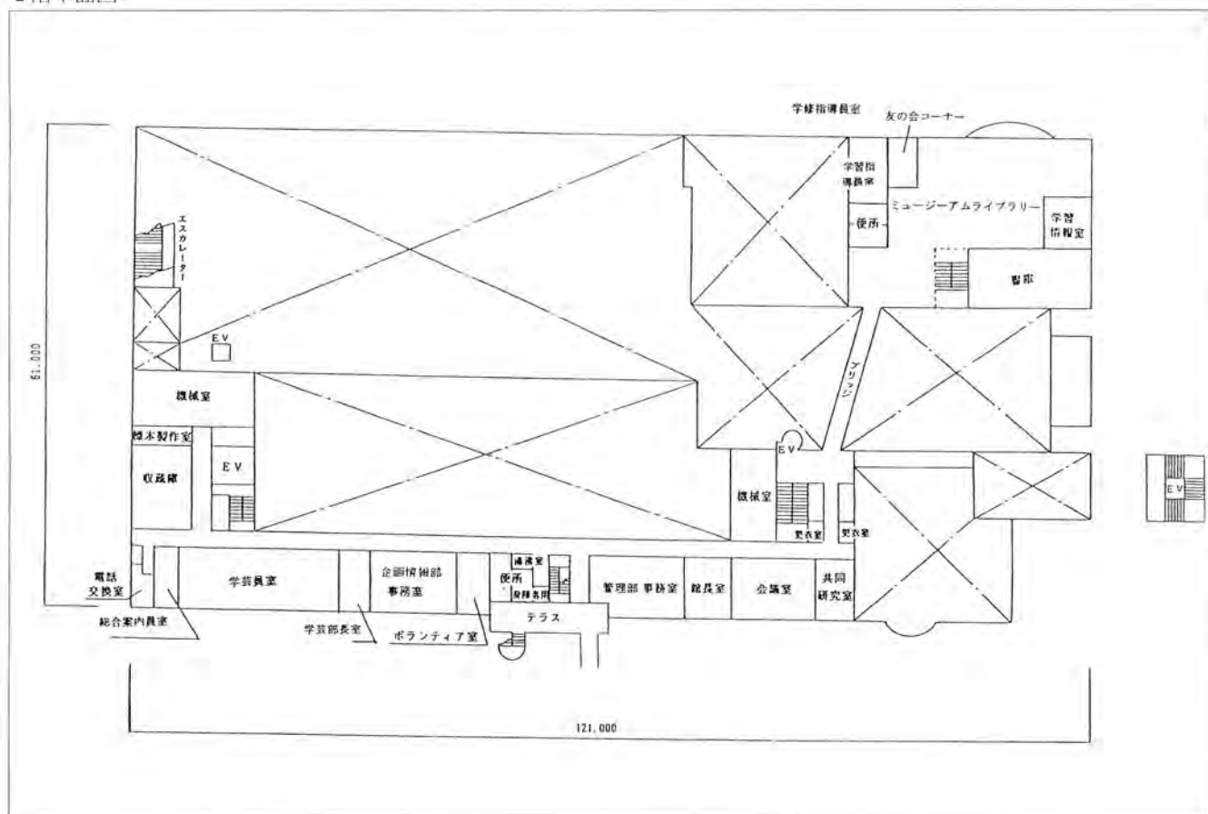
2 階平面図
