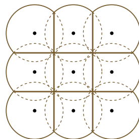
図4 正三角形・正方形の頂点に穴をあけたときにできるもよう（上から見た図）。円同士がぶつかったと、その交点を結んだ直線があらわれる。
