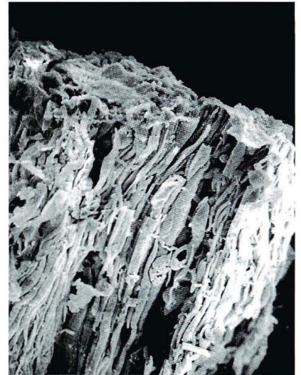
図8 風化した火山灰。おもに繊維状に伸びた気泡からなるが、小さな丸い気泡もある。火砕流の地層上部（座間市栗原），写真の左右幅0.15 mm.
