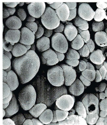
図4 風化している軽石。紙面手前側には鉱物が付着していたらしく、気泡の末端部が見えている。火砕流の地層上部（海老名市大谷）、写真の左右幅0.5 mm。
