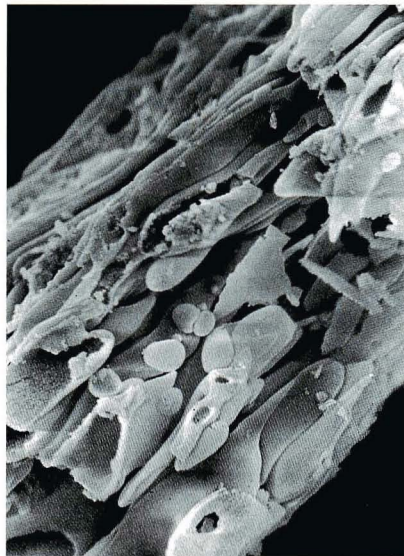
図7 風化した火山灰。大きな気泡は伸びた状態であるが、小さな丸い気泡もある。火砕流の地層上部（海老名市大谷），写真の左右幅0.15 mm.
