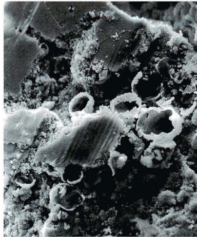
図6 卵の殻のように見える風化物。背面は鉱物、平滑な手前の面も鉱物が付着していた跡。鉱物にはさまれた火山ガラスの気泡が残ったと考えられる。火砕流の地層上部（大和市中鶴間），写真の左右幅0.15 mm.
