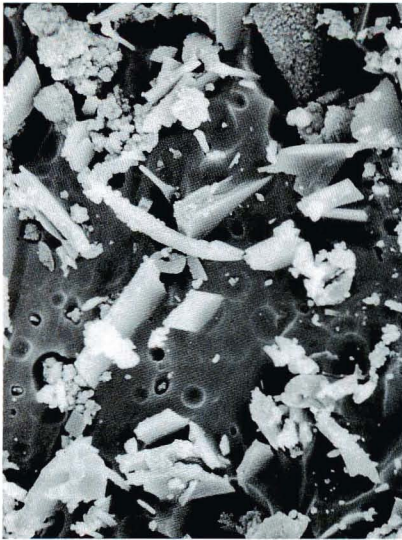
図5 失われていく火山ガラス。飛び出ているのは鉱物（斑晶）。浅い皿状の凹面は気泡の一部ではなく、風化でできたものである。火砕流の地層上部（海老名市大谷），写真の左右幅0.5 mm.
