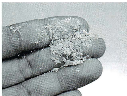
図2 風化している軽石。火山ガラスは失われ、もはや粒としては取り出せない。図1に相当する部分だが、色もオレンジ色になっている。東京軽石層上部（平塚市上吉沢）。
