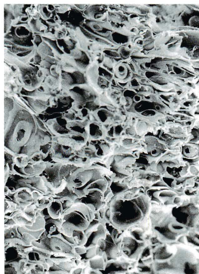
図3 あまり風化していない軽石。人為的に割って新鮮な部分を出したもの。東京軽石層中部（横浜市泉区新橋町）、写真の左右幅0.6 mm。
