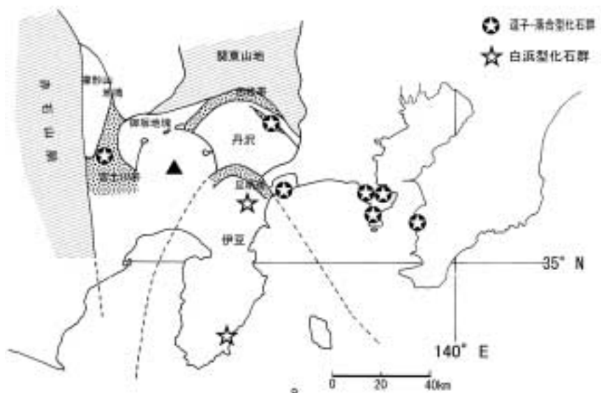
図 8. 南部フオッサマグナ地域における中新世後期～鮮新世前期の逗子一落合型貝化石群の地理的分布 (鎮西・松島, 1987).
