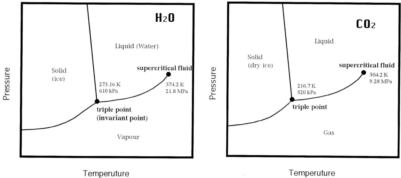
図9. H 2 O と CO 2 の模式的状態図.
