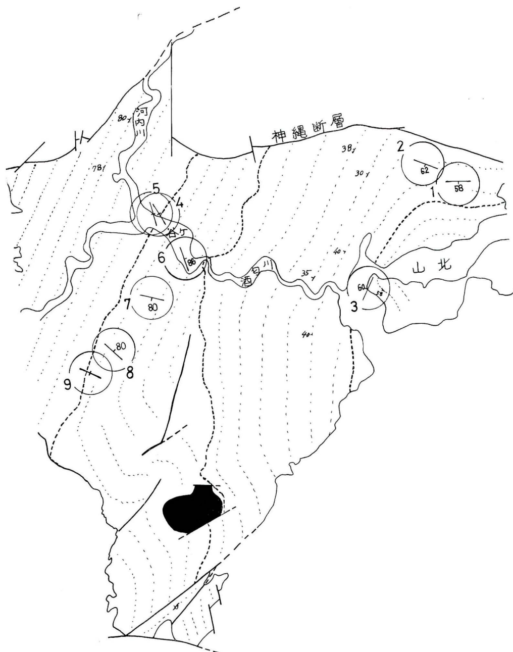
図 1. 足柄層群の構造図と計測した岩脈の分布図
