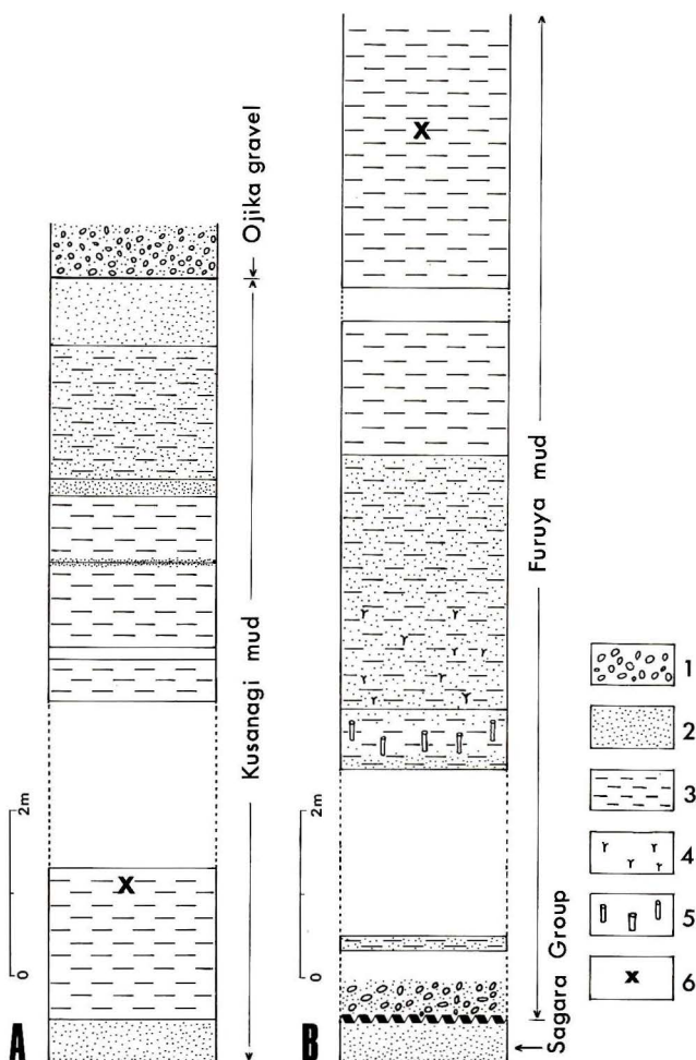
図2. 草薙泥層(A)および古谷泥層(B)の地質柱状図。 1, 砂礫岩; 2, 砂岩; 3, シルト岩; 4, 泥炭; 5, サンドパイプ; 6, 鉗脚鋏部化石産出地点。(土・池谷(1970, 1971)の調査資料より作成)。
