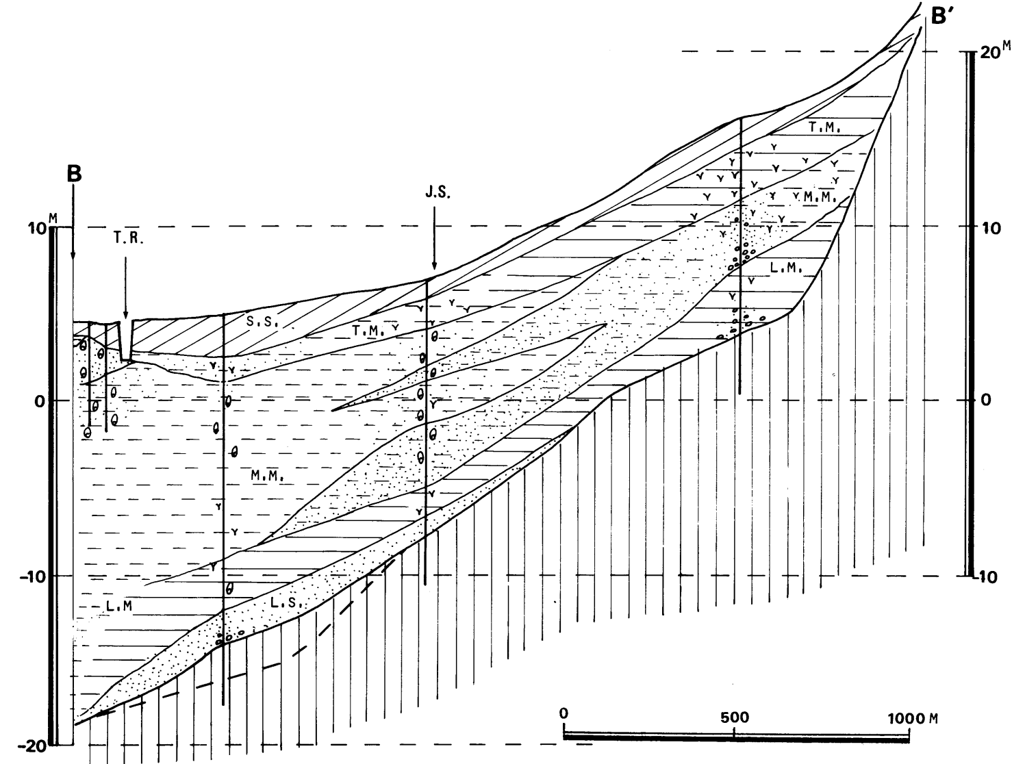
第 2 - 5 図 池子川沿の B - B' 地質断面図
