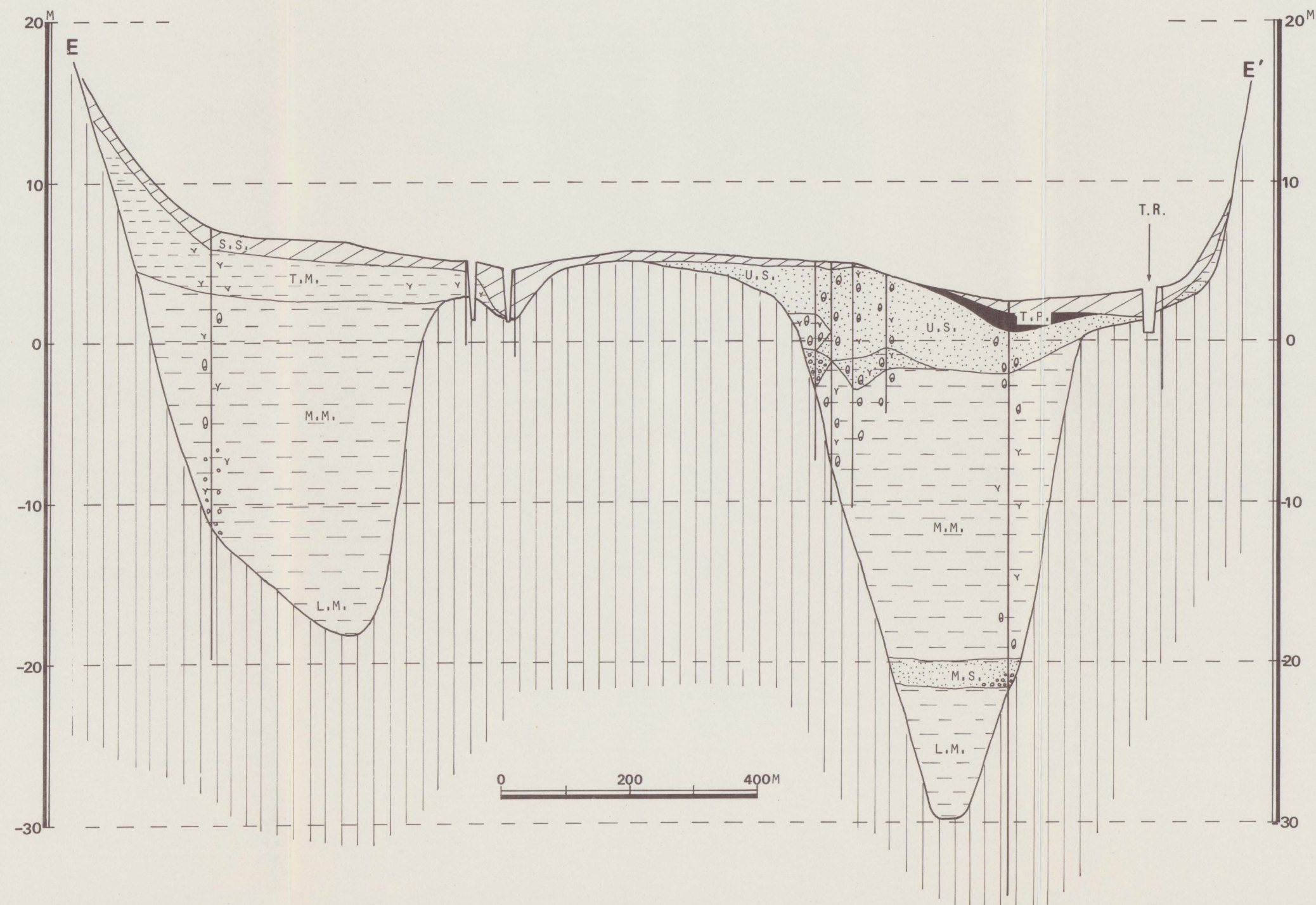
第 2 - 8 図 逗子貝層の E - E' 地質断面図
