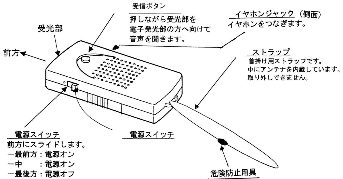
図4. 「受信機」(タイプ1).
