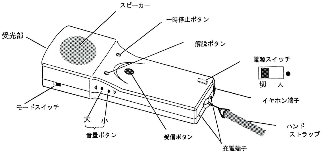
図5. 「受信機」(タイプ3).
