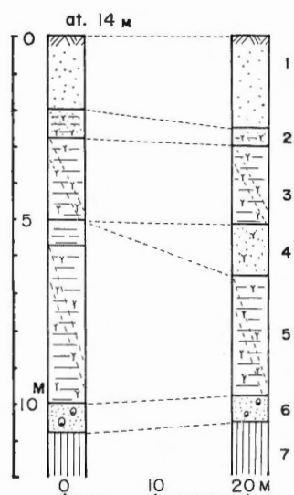
第5図 新吉原橋のボーリング柱状図(海拔:14m)
