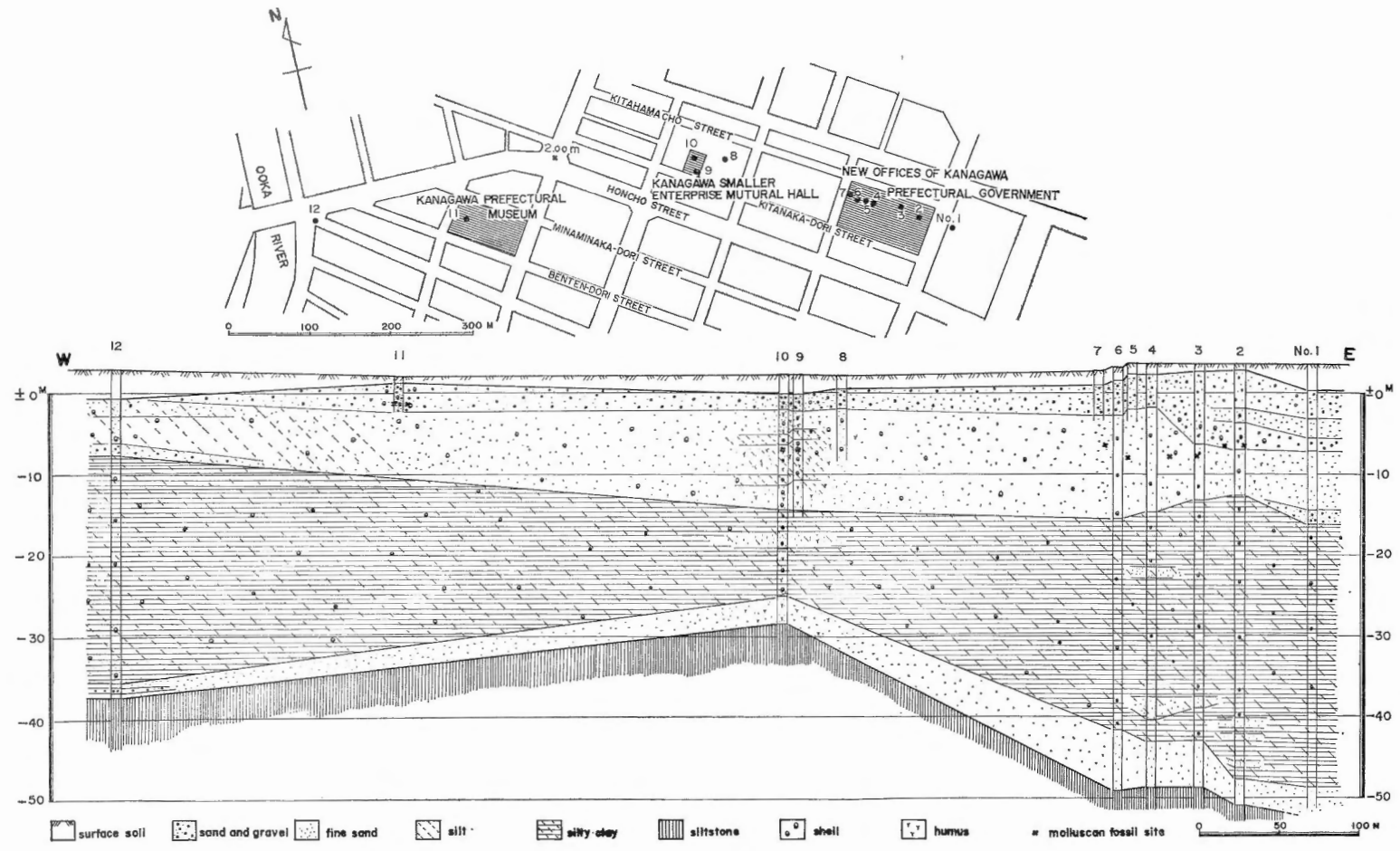
第3図 横浜市内A地域の沖積層の層序断面とボーリング位置図 Fig. 3 Site of boring and section of sedimentary facies of alluvial deposits of A area in Yokohama City.
